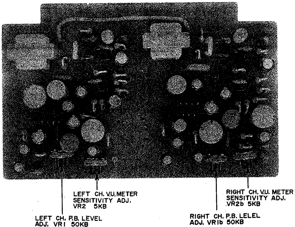
Fig. 20 P.B. AMP. P.C. BOARD (FACE SIDE)
