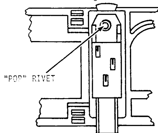
SWITCH P.N. 187000
